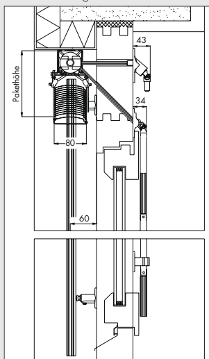
Schnittzeichnung S80
