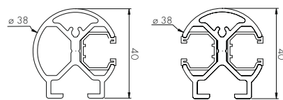
Einzel- und Doppelführungsschiene
