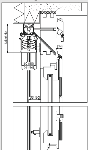
Schnittzeichnung K80
