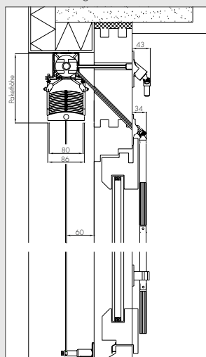
Schnittzeichnung F80
