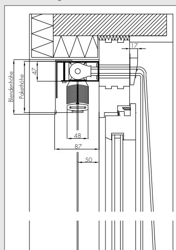
Schnittzeichnung
